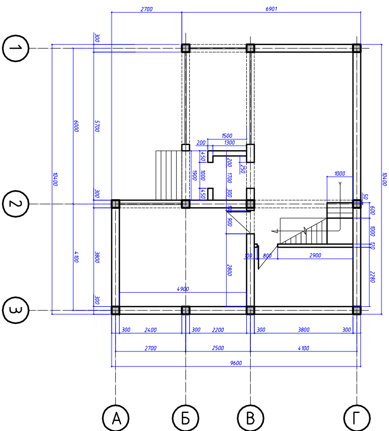
План 1 этажа (вариант 1)
