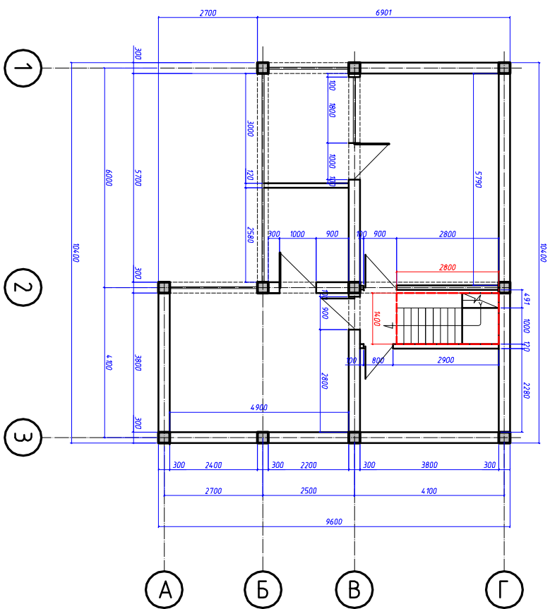
План 2 этажа (вариант 2)
