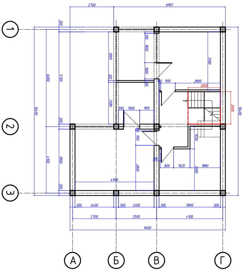
План 2 этажа (вариант 1)
